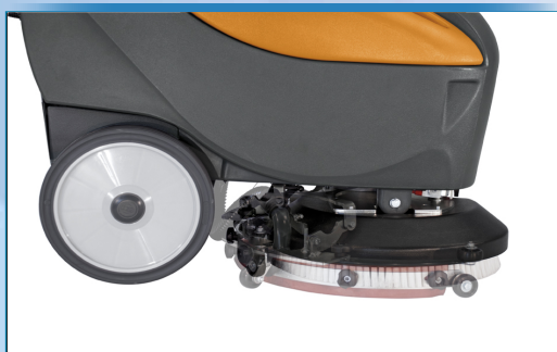
MEEDRAAIENDE ZUIGMOND
